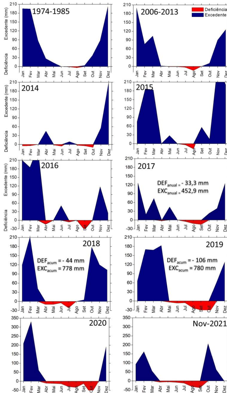
Figura 8: Balanço hídrico mensal sequencial (THORNTHWAIT E MATHER, 1955) no período de 1974-1985, 2006-2013, para os anos de 2014, 2015, 2016, 2017, 2018, 2019, 2020 e 2021 para a região do Sul de Minas, Muzambinho.
